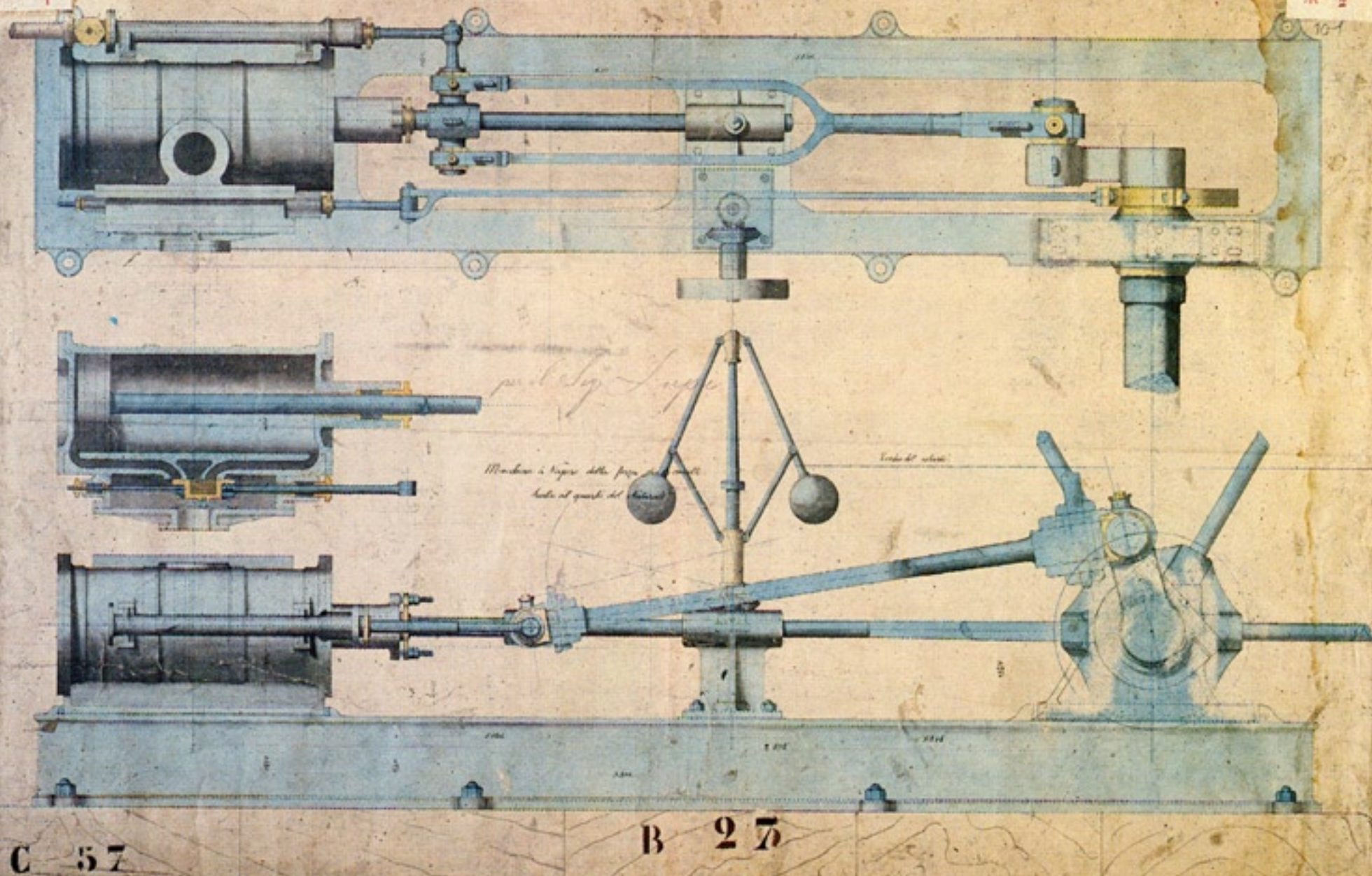
Disegno macchina a vapore. 1880 Fondazione Ansaldo, Genova
