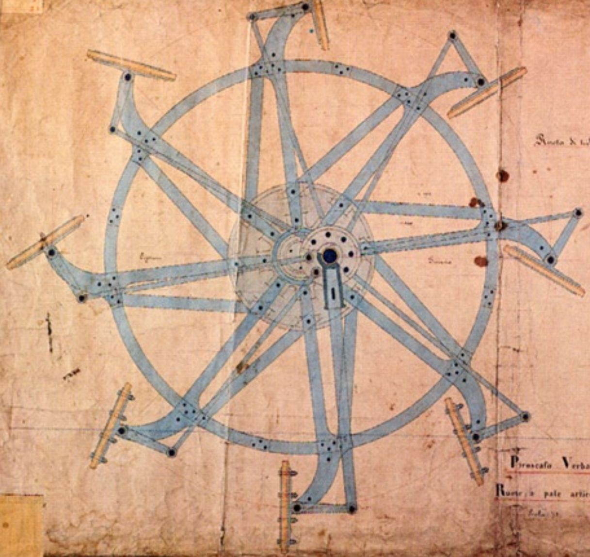
Disegno ruota piroscavo Verbano. 1856 Fondazione Ansaldo, Genova
