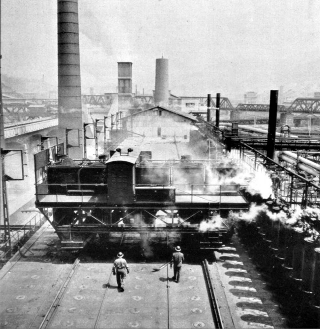
Acciaierie di Cornigliano. I forni coke. Fonte: Rivista di Cornigliano 1957 n.1 presso Fondazione Ansaldo, Genova - www.storiaindustria.it
