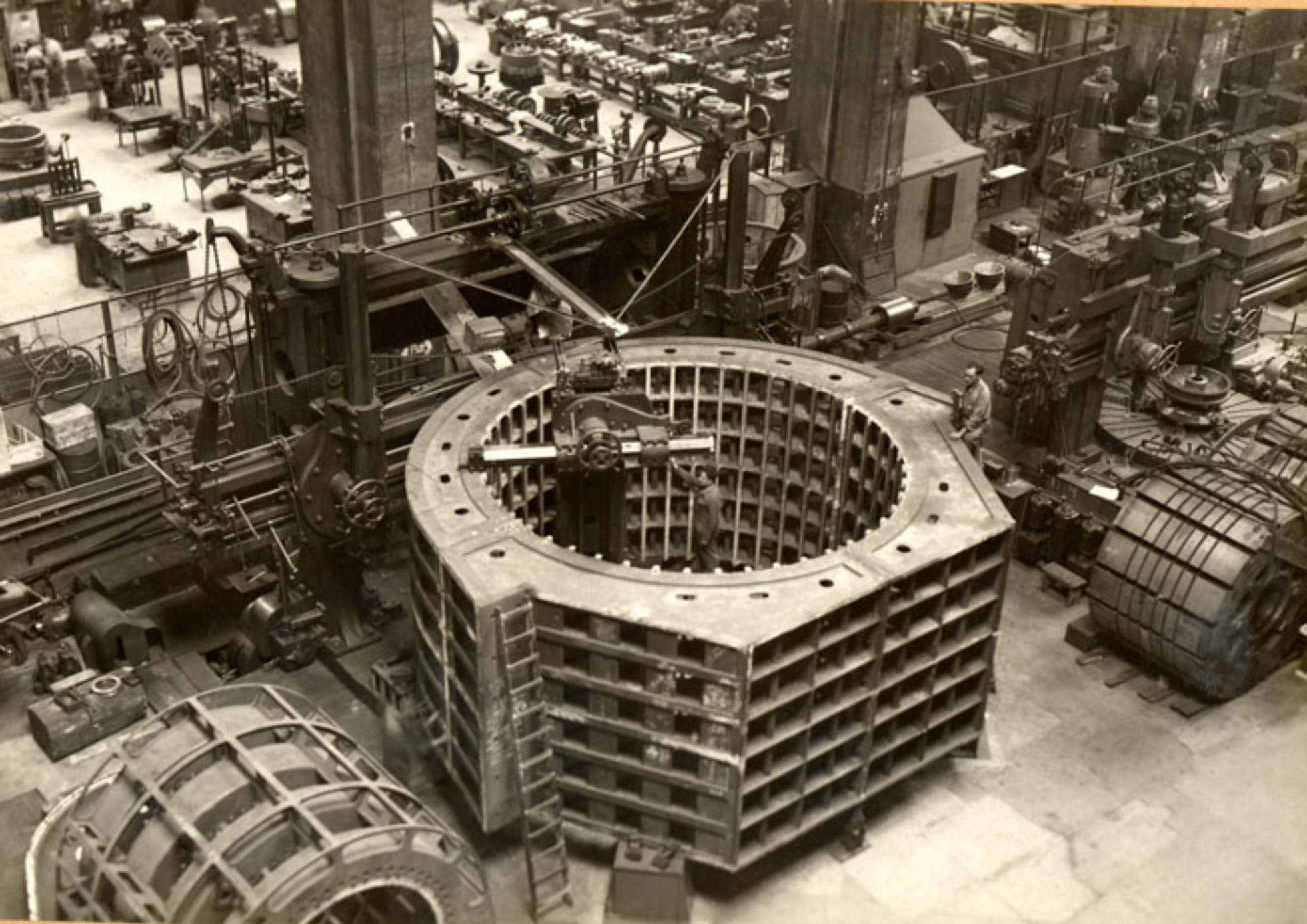
Lavorazione di un alternatore all'interno dello Stabilimento Elettrotecnico Ansaldo. Genova Cornigliano, 1941 Fondazione Ansaldo, Genova
