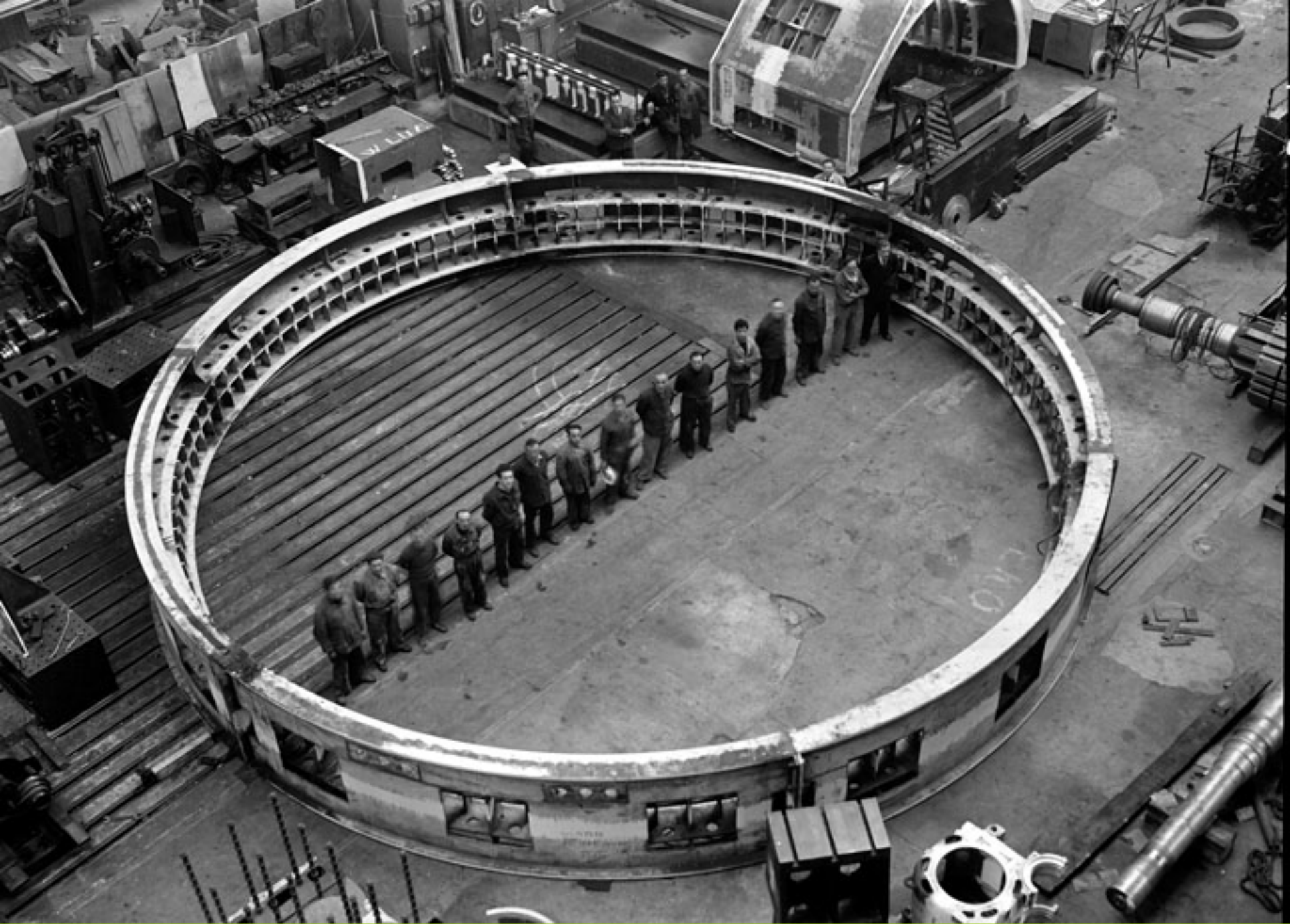
Stabilimento Elettrotecnico Ansaldo. Lavorazione alternatore. Genova Cornigliano, 1953 Fondazione Ansaldo, Genova
