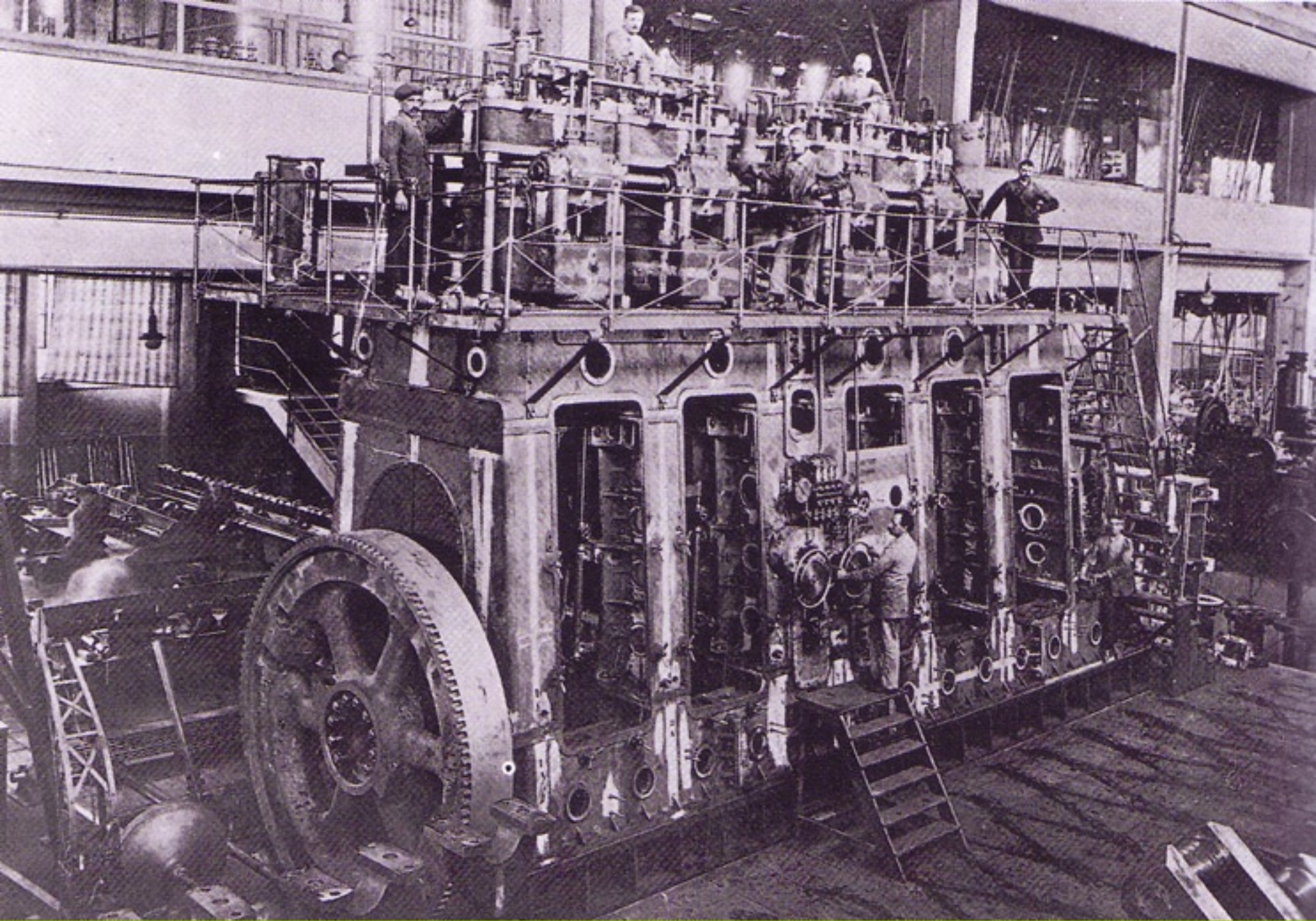
Un motore diesel. cantieri Officine Savoia di Cornigliano (Genova), 1920 Fondazione Ansaldo, Genova
