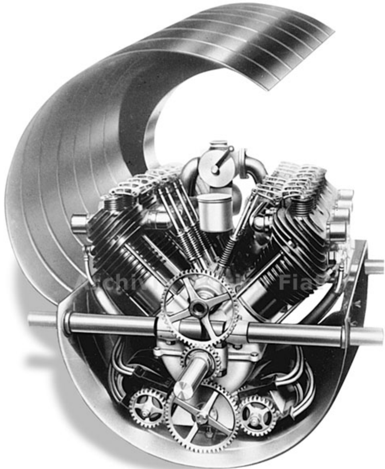
Il 1° motore per aviazione realizzato dalla Fiat, l'SA 8/75, 8 cilindri a V da 50 Cv. 1908 Archivio Storico Fiat, Torino
