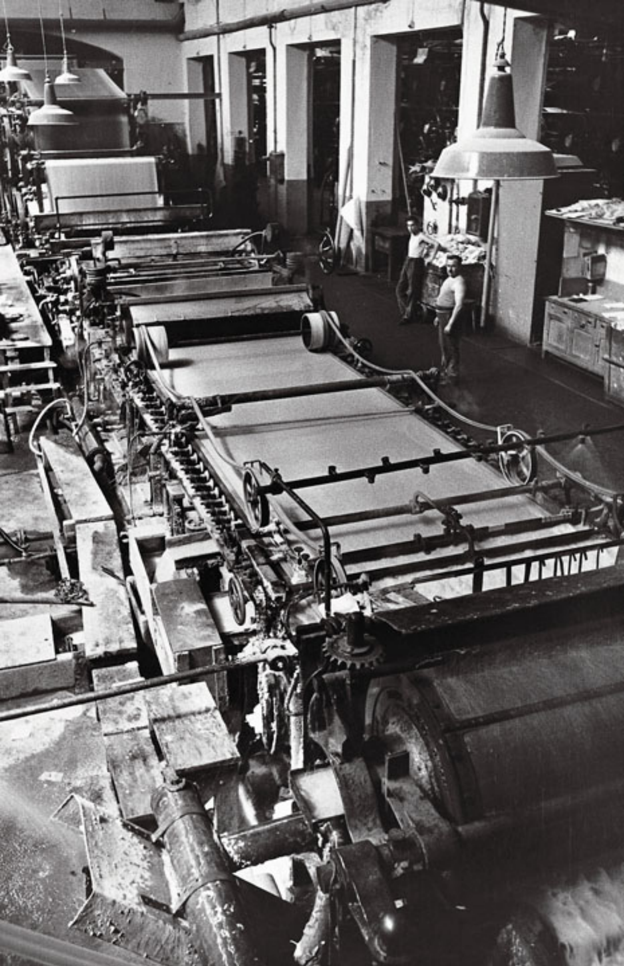
La "continua uno" dello stabilimento Burgo. Verzuolo (CN), 1906 Archivio Storico Burgo Group, San Mauro Torinese (TO)
