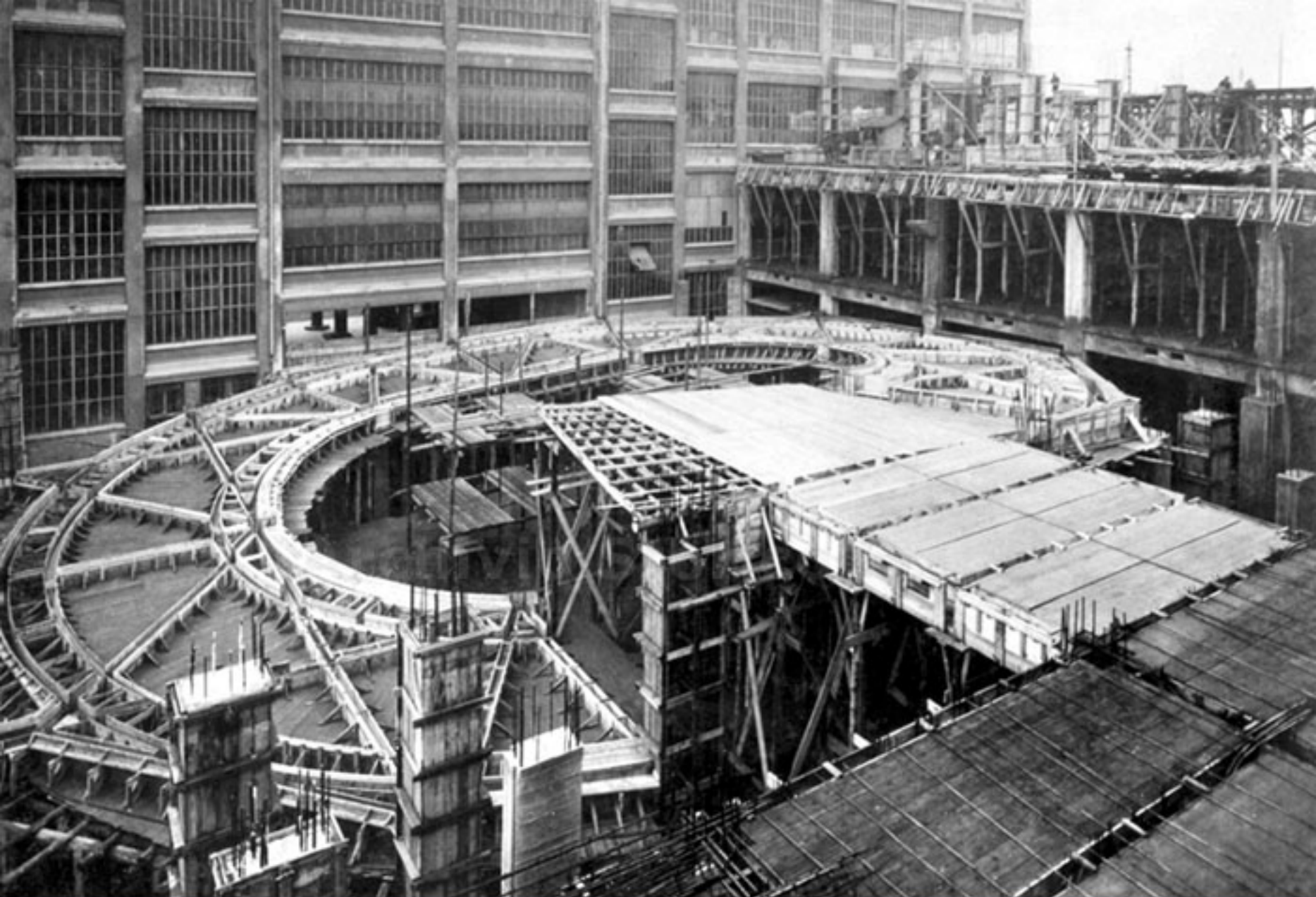
Armatura del primo piano della rampa nord del Lingotto, ampliamento della Sezione automobili. Torino, 1925 Archivio Storico Fiat, Torino
