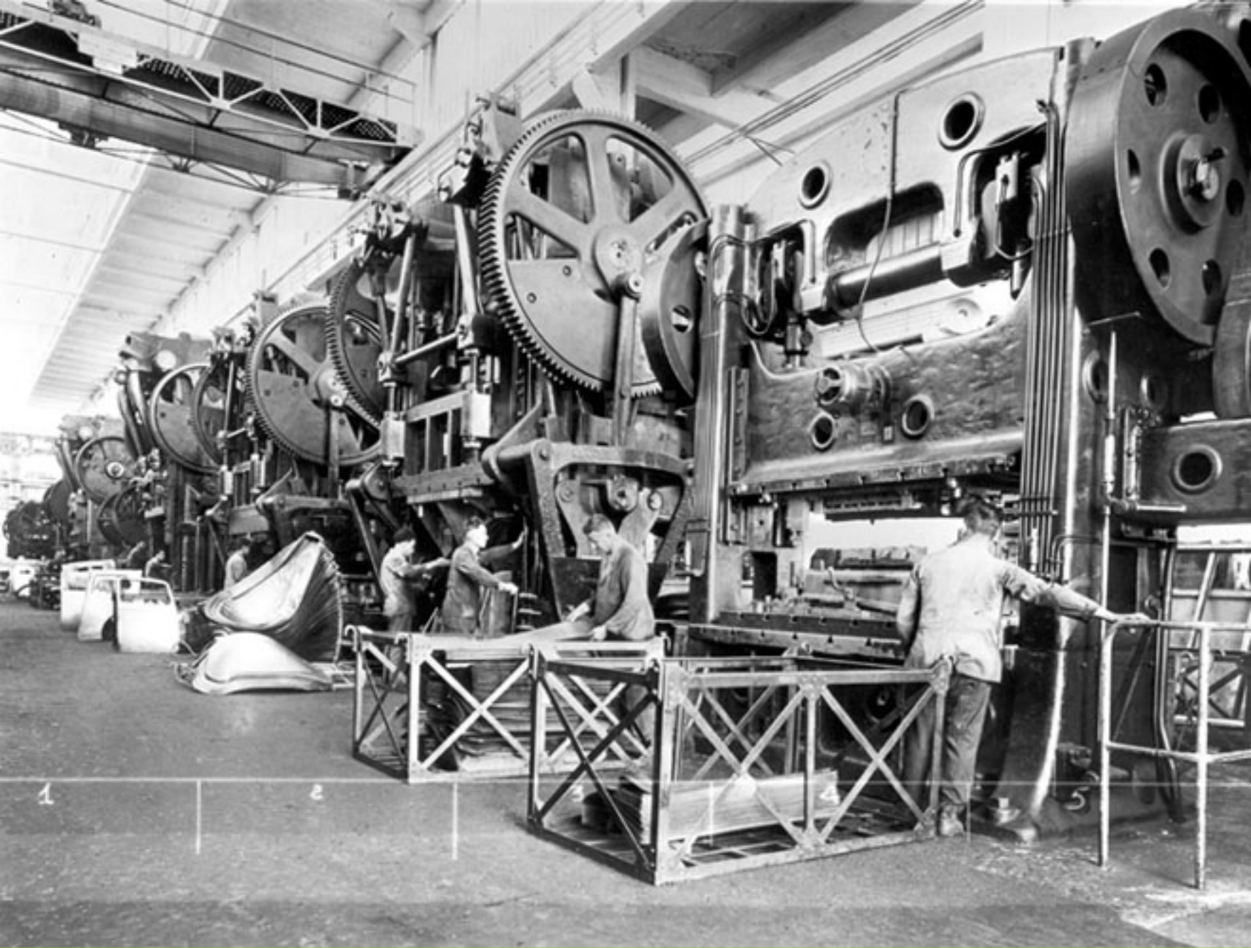
Stabilimenti FIAT del Lingotto. Grandi presse per lo stampaggio delle fiancate. Torino, 1933 Archivio Storico Fiat, Torino
