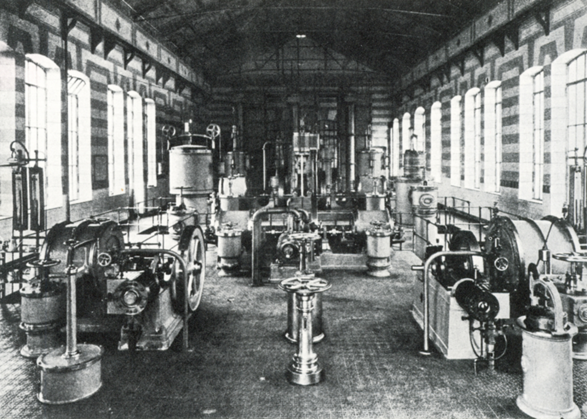
Sala macchine dell'officina Vanchiglia della Società Consumatori Gas-Luce. Torino, 1902-1908 Archivio Storico Italgas, Torino
