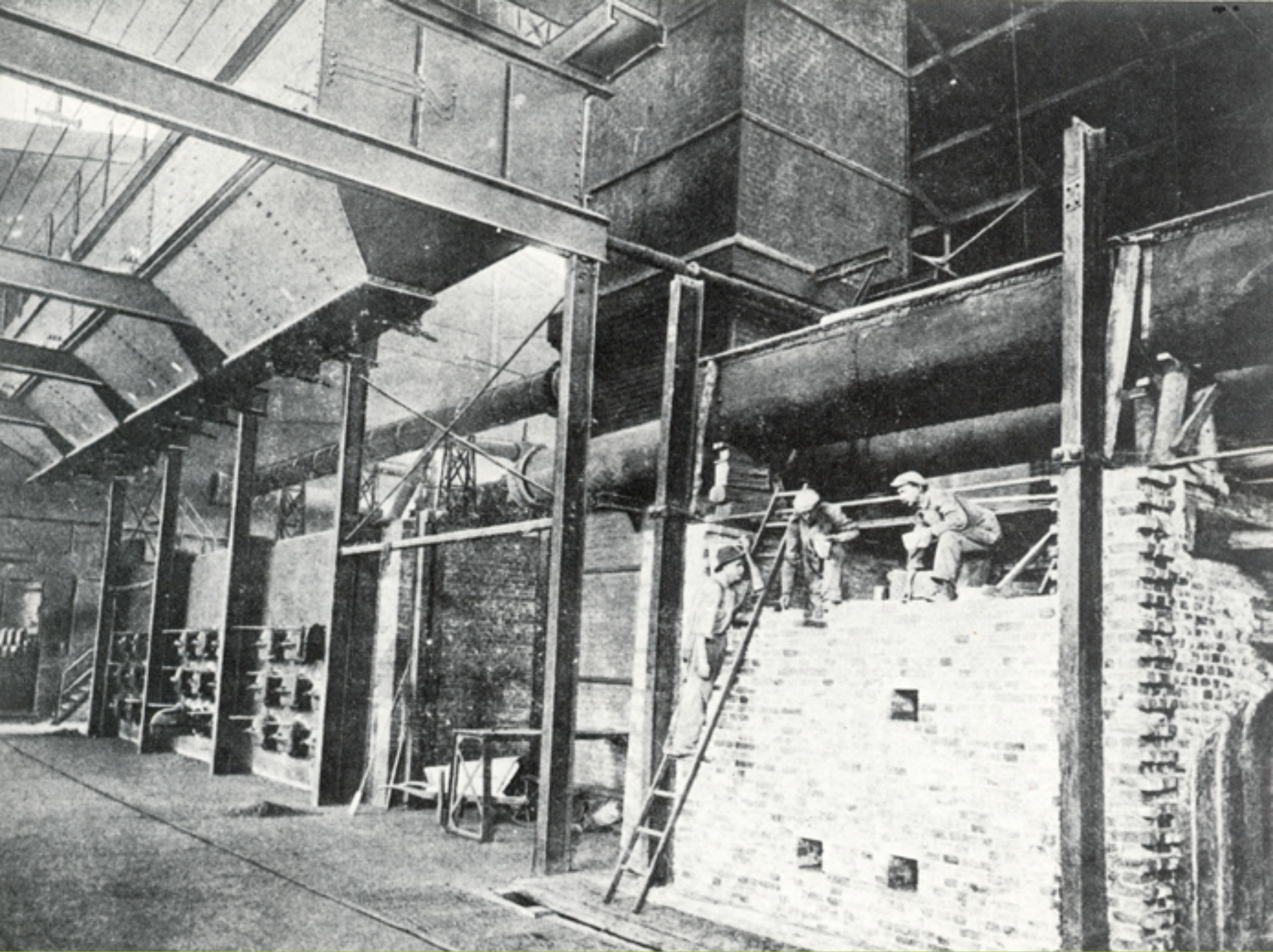
Costruzione di un gasogeno a legna, Torino 1917-1918 Archivio Storico Italgas, Torino
