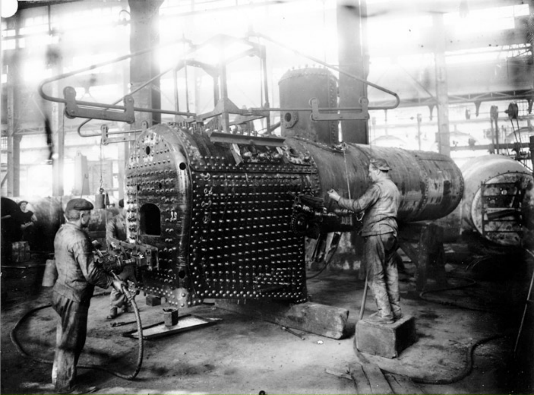
Caldia per locomotiva. 1902 circa Fondazione Ansaldo, Genova
