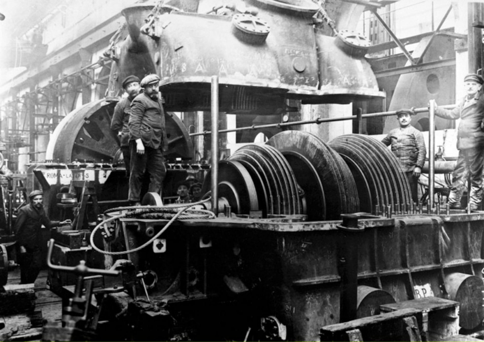
Lavorazione turbina. Stabilimento Meccanico Ansaldo. Genova Sampierdarena, 1926 Fondazione Ansaldo, Genova
